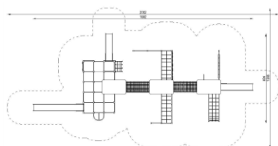
Rzut urządzenia wraz ze strefą funkcjonalną:
