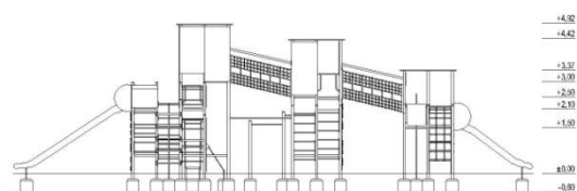
Widok urządzenia:
